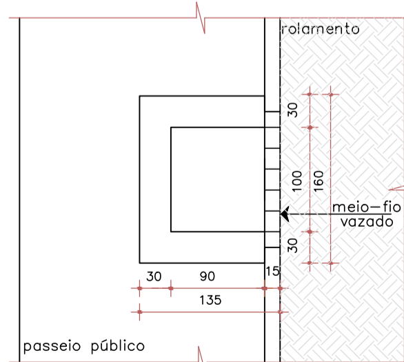
DETALHE BOCA DE LOBO Escala 1/50
