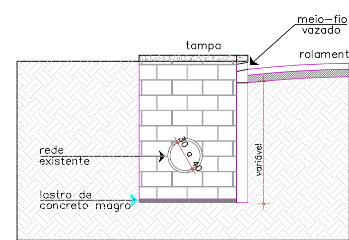
CORTE TRANSVERSAL Escala 1/50
