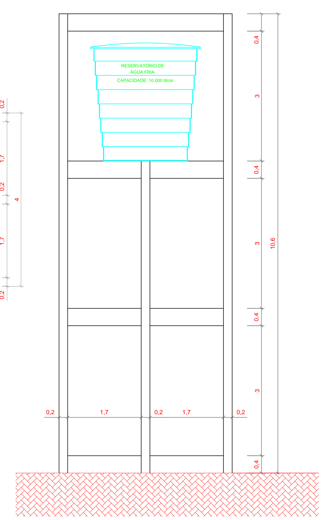
2 CORTE A-A' ESCALA 1/50
