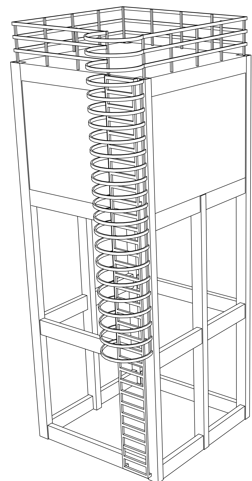
3 ISOMÉTRICO ESCALA 1/50
