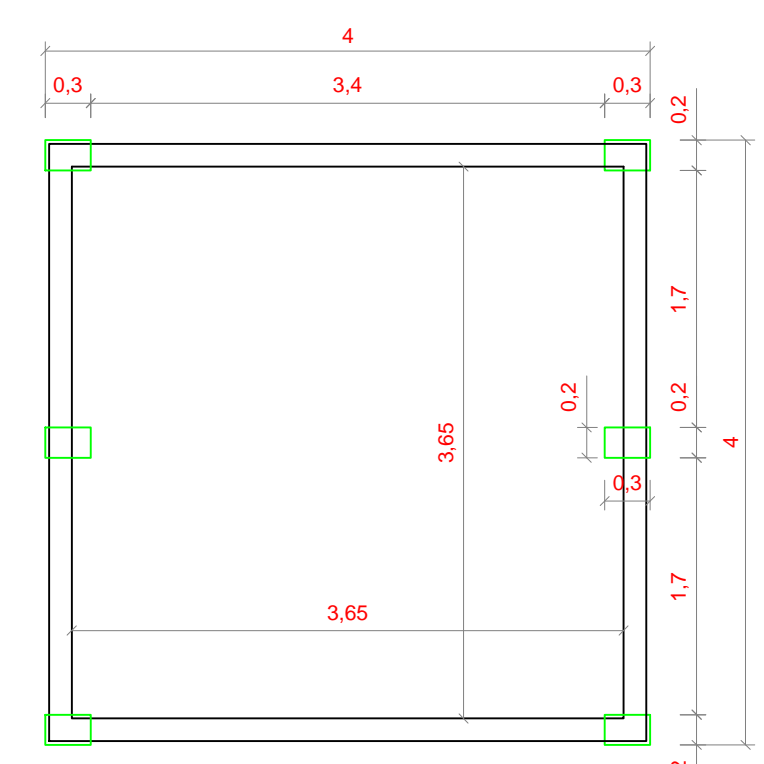
1 PLANTA BAIXA ESCALA 1/50
